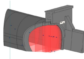
Abb. 3.1.12.-3: Luftraum Tunnel im Schnitt
