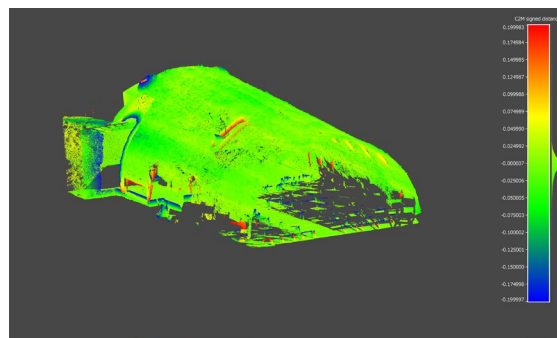
Abb. 3.1.20-8: Abstand Modell zu Punktwolke
