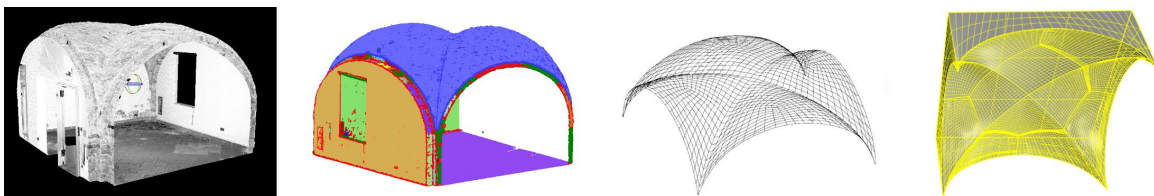
Abb. 3.1.22-3: Automatisierung zur Erstellung BIM konformer Gewölbemodelle mit hoher verformungstreue, Freeform4BIM, TLS Tagung Fulda 2023
