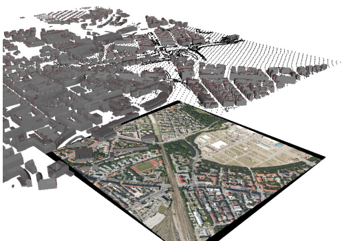
Abb. 3.1.16-3: Bestandsdaten des Geoportal Bayern nach Transformation ins PKS
