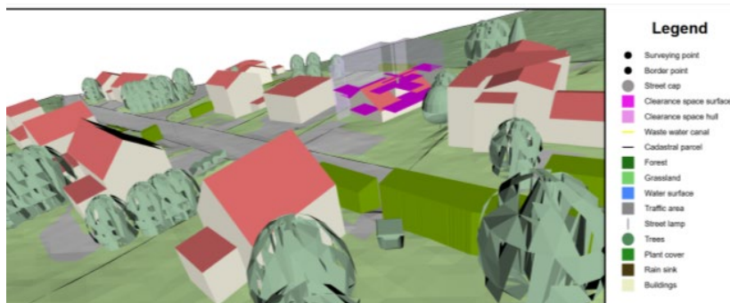
Abb. 2.6.1-2: Visualisierung eines dreidimensionalen Lageplans nach der CityGML SitePlan ADE (Müller 2021).
