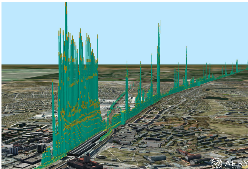
Abb. 3.2.4-3: Verknüpfung BIM-basierter Ökobilanzierung mit GIS ermöglicht Visualisierung im Kontext der Umgebung (Quelle: AFRY)
