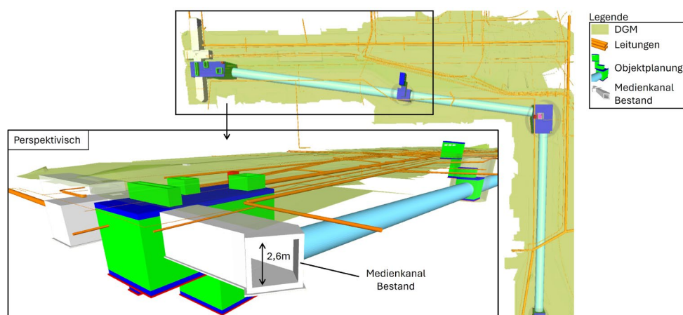
Abb. 3.1.14-2: Draufsicht des bestehenden und beplanten Medienkanals mit perspektivischem Detailausschnitt der Fachmodelle IBW, DGM, INF, LAA (Urheberschaft: BlmA)
