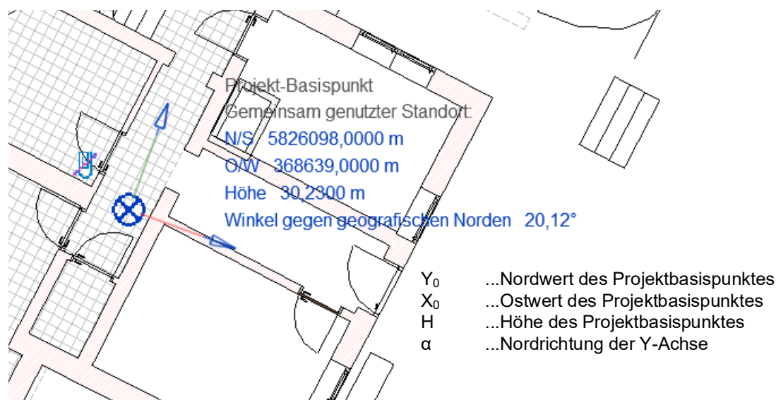
Abb. 2.2-5: Georeferenzierter Projektbasispunkt in der BIM Autorenssoftware Autodesk Revit.
