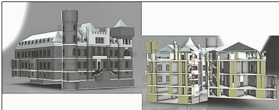
Abb. 3.1.17-2: IFC- Modell des Schlosses (links) und Schnitt durch das Modell (rechts)
