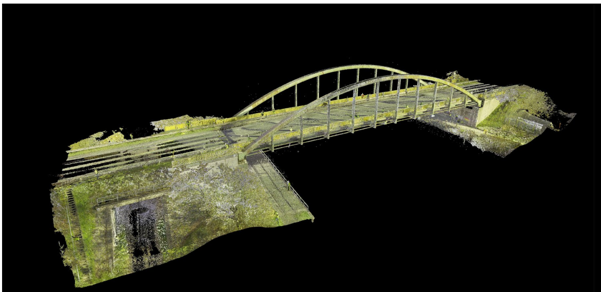
Abb. 3.1.13-2: Punktwolke der Drewer Brücke (©BIM.Ruhr)
