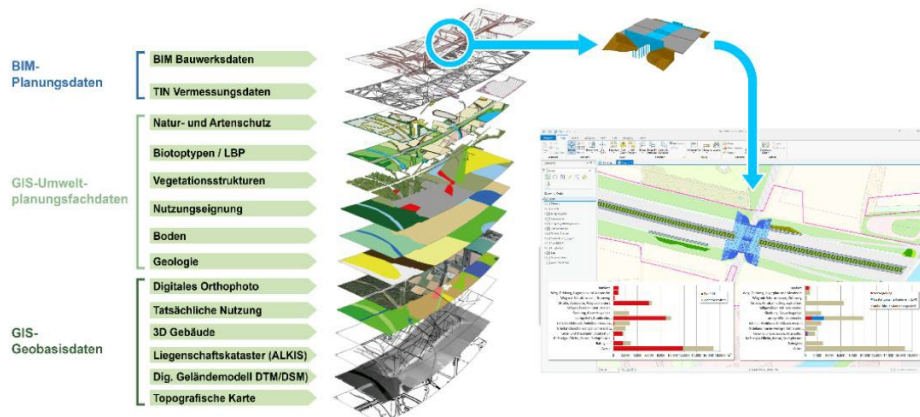
Abbildung 3.2.3-112: Das Bauwerk im räumlichen Gesamtkontext, mit Geobasis- und Fachdaten im GIS und mit Prüfung der Umweltwirkungen (psu).
