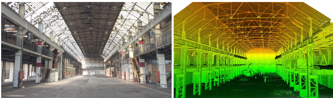
Abb. 3.1.11-2: Innenansicht der Industriehalle vor den Revitalisierungsmaßnahmen (links: Fotografie, rechts: Punktwolke)
