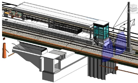
Abb. 3.1.9-3: Revit-Modell.
