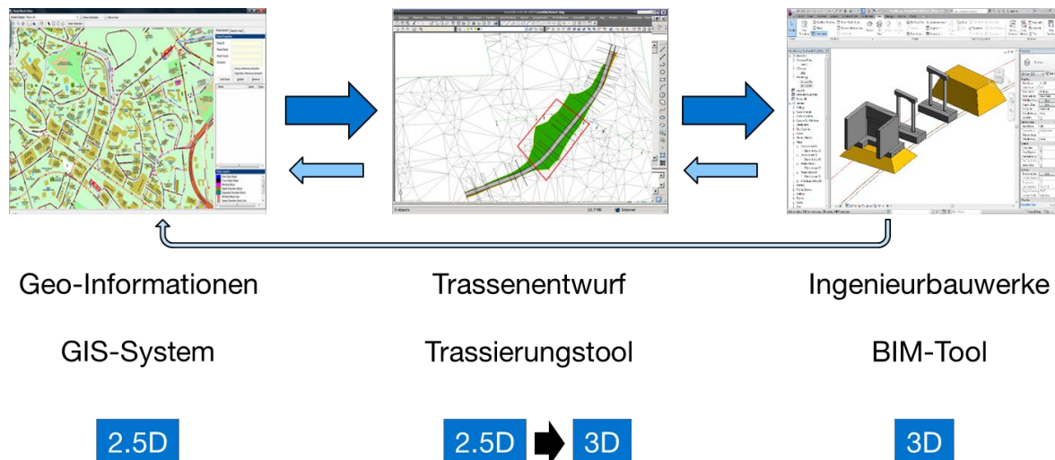
Abb. 2.1-22: Eine typische digitale Kette im Infrastrukturbau, bei der unterschiedliche Softwaresysteme mit unterschiedlichen Philosophien und Modellierungsparadigmen zusammenspielen müssen.
