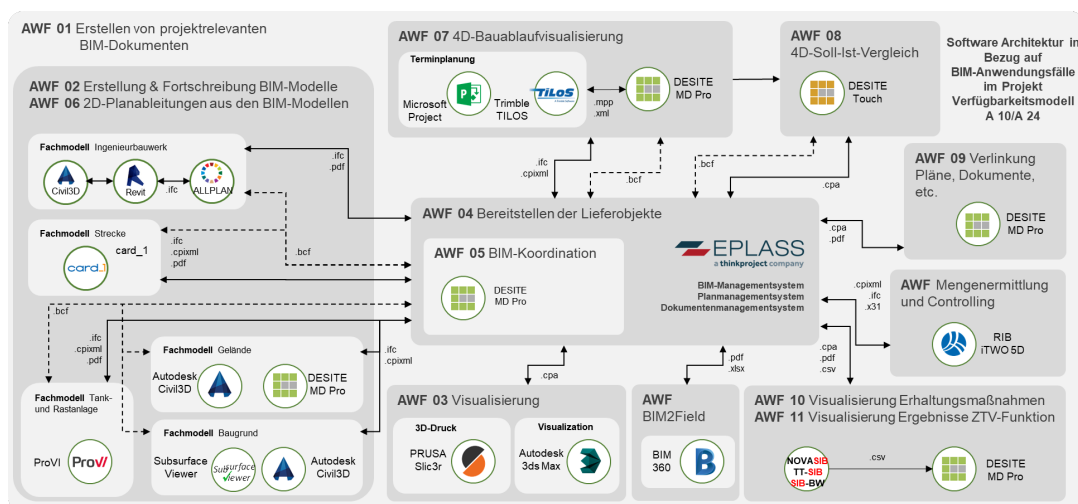
Abb. 3.1.6-2: Software Architektur im Projekt „Verfügbarkeitsmodell A 10/A 24“.
