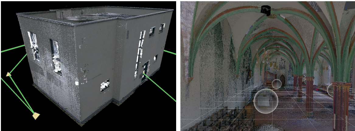
Abb. 3.1.8-2: Links: Punktwolke der Stadtvilla visualisiert in Leica Cyclone Register 360. Rechts: Punktwolke des gotischen Klosterbaus visualisiert in Autodesk ReCap.
