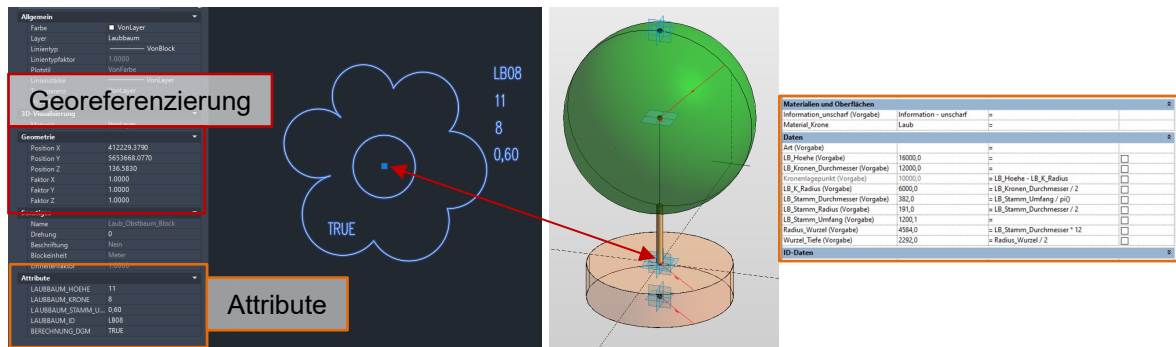
Abb. 4.4-4: CAD-Integration im CityBIM-Plug-in.
