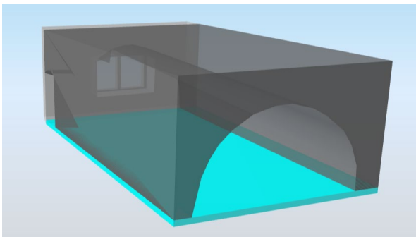
Abb. 3.1.20-7: Bauteile eines Raums
