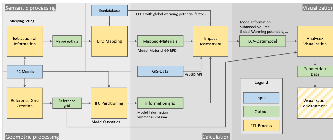
Abb. 3.2.4-2: Prozessarchitektur der von AFRY entwickelten Methode zur Ökobilanzierung mit den Teilprozessen ‚Extraction of Information‘, ‚EPD Mapping‘, ‚Reference Grid Creation‘, ‚IFC Partitioning‘, ‚Impact Assessment‘ und ‚Analysis/Visualization‘ (Quelle: AFRY)
