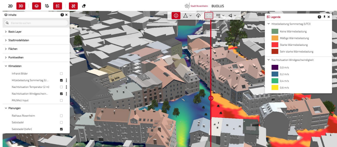
Abbildung: Integration von BIM-Modellen in den Stadtmodellkontext als Basis für Klimauntersuchungen am Beispiel des Forschungsprojektes BUOLUS zum Salzstadel in Rosenheim.
