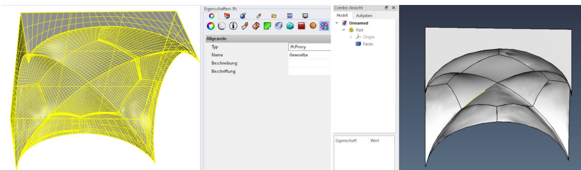
Abb. 3.1.22-4: BIM konforme Attribuierung von CAD-Objekten mit Freiformflächen zur Erstellung von IFC Objekten, Freeform4BIM, TLS Tagung Fulda 2023
