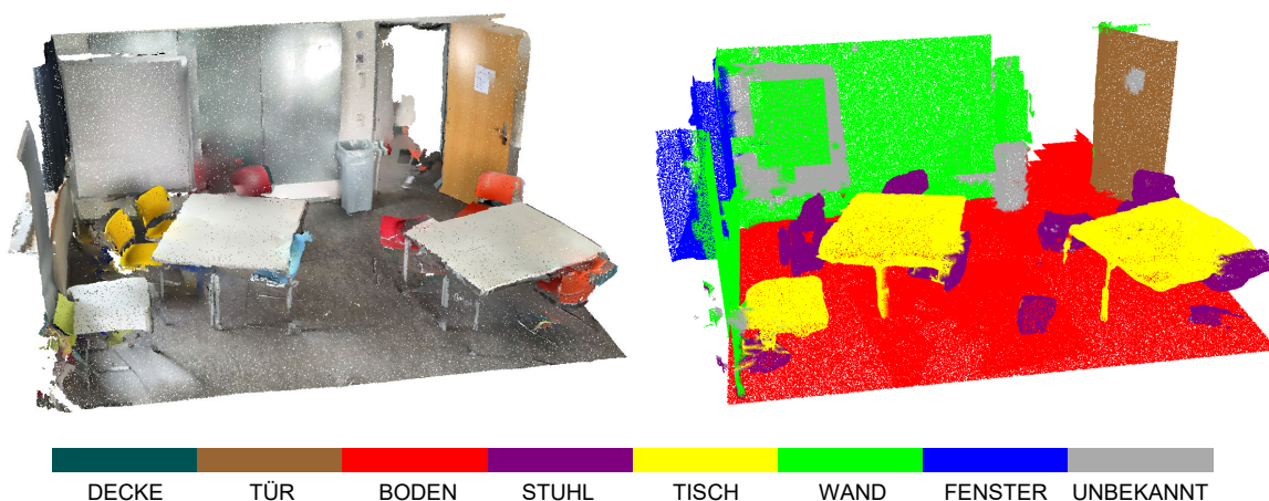
Abb. 3.1.5-2: Visualisierung der RGB-texturierten (links) und in Echtzeit klassifizierten (rechts) 3D-Punktwolke durch die entwickelte AR-Anwendung, erfasst mit einem Apple iPhone 12 Pro.
