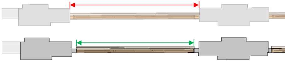
Abb. 3.1.11-4: Interpretationsansätze eines Fensterelements im Grundriss (oben: Fensterrahmen zu breit angenommen, unten: Konstruktiv korrekte Zuordnung).
