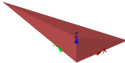
Abb. 2.2-6: Volumetrischer Koordinationskörper für die Prüfung der Georeferenzierung (Schapke 2020).
