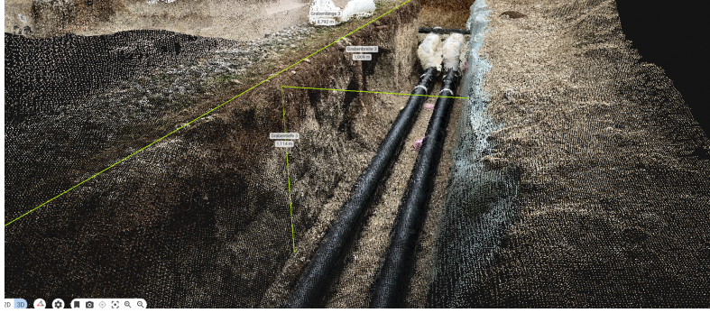
Abb. 3.1.19-4: Ermittlung von Grabenbreite, -tiefe und -länge für die Abrechnung
