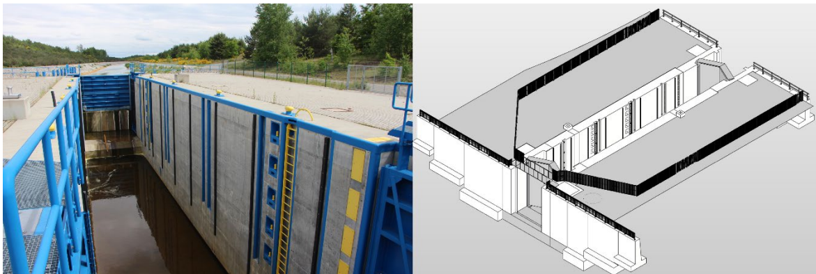
Abb. 3.1.4-1: Blick in die Schleusenkammer (Foto: Palme), BIM-Modell der Schleuse.
