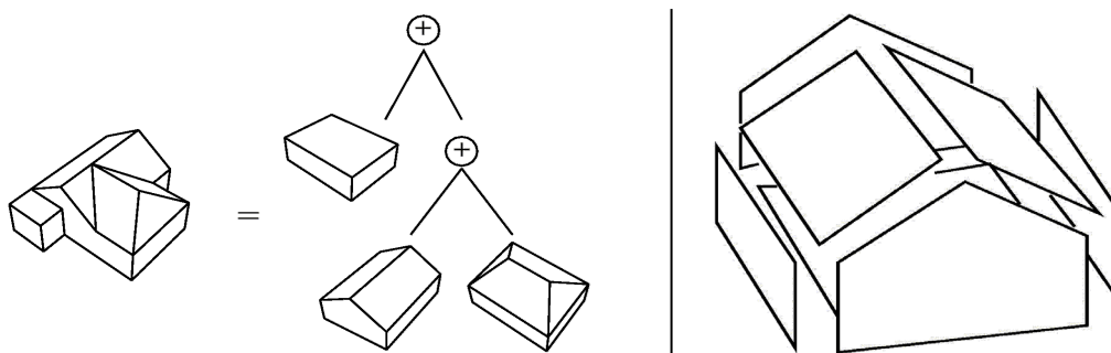
Abb. 2.3-6: Geometrirepräsentation in BIM durch parametrische Elemente, CSG oder Sweep und logischer Verknüpfung der Grundelemente (links) und in GIS durch Akkumulation aller umschließenden Begrenzungsflächen (B-Rep) (rechts). Adaptiert von (Kolbe & Plümer 2004).
