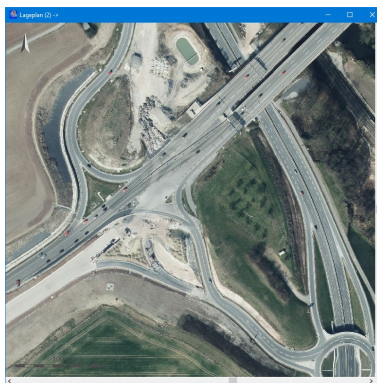
Abb. 3.2.2-1: Luftbild mit 20 cm Bodenauflösung.
