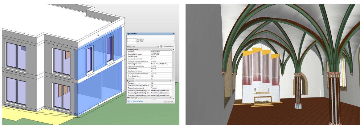
Abb. 3.1.8-3: Links: BIM-Modell der Stadtvilla im Bauhausstil mit selektierter Wand im normierten Rohbaumaß (inkl. Putzabzug), visualisiert in der BIM-Autorensoftware Revit von Autodesk. Rechts: BIM-Modell des gotischen Klosterbaus mit Deckenkonstruktion bestehend aus Bündelpfeiler, Rippen und Kappe, visualisiert in der BIM-Autorensoftware Allplan von Nemetschek.
