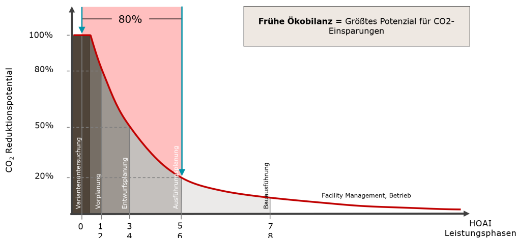
Abb. 3.2.4-1: Potenzial zur Reduktion von Treibhausgas-Emissionen im Projekterlauf (Quelle: AFRY)
