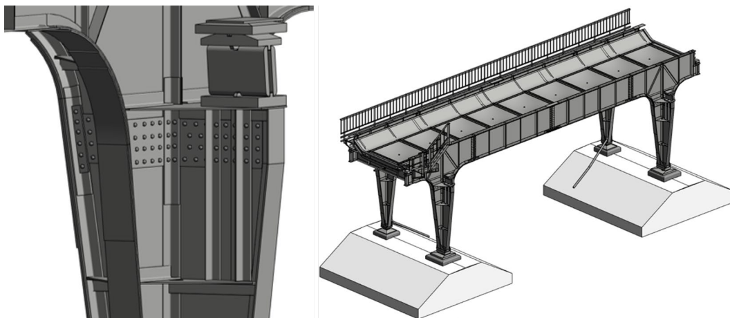
Abb. 3.1.10-2: LOD-400-Bestandsmodell des Eisenbahnviadukts.
