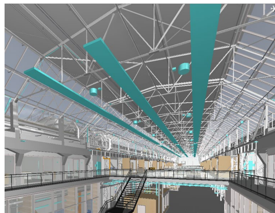
Abb. 3.1.11-3: Innenansicht des Bestandsmodells mit eingearbeiteter Ausführungsplanung der Architekten und TGA-Planer.
