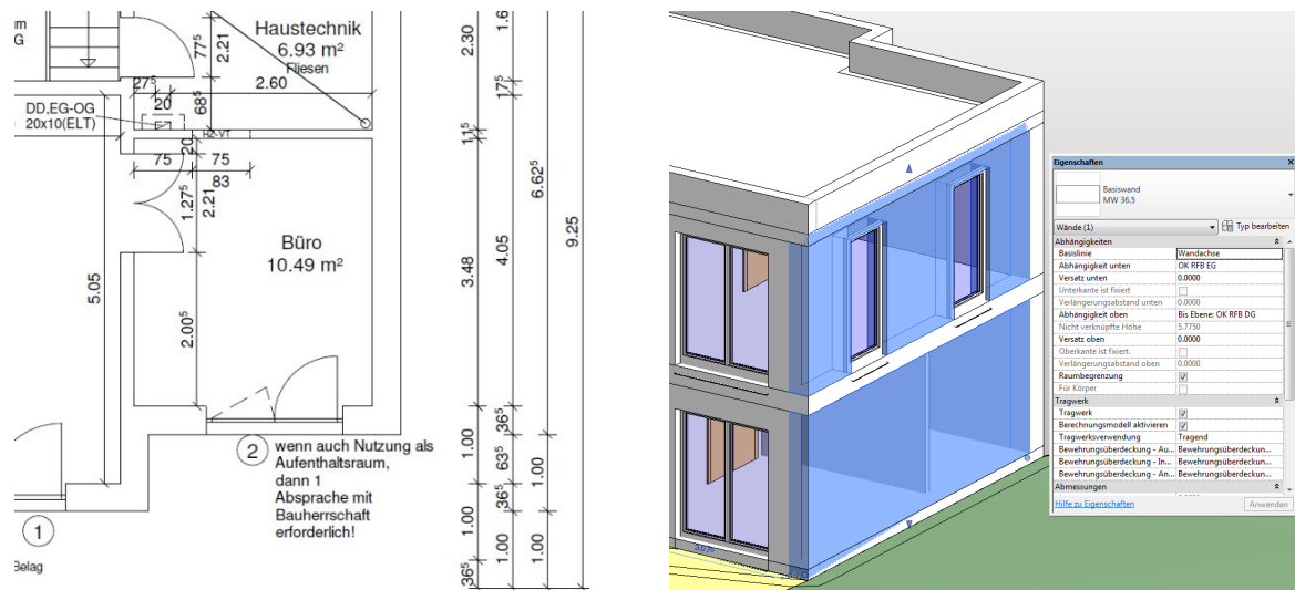
Abb. 2.3-1: Vergleich CAD-Zeichnung (links) und BIM-Modell (rechts).
