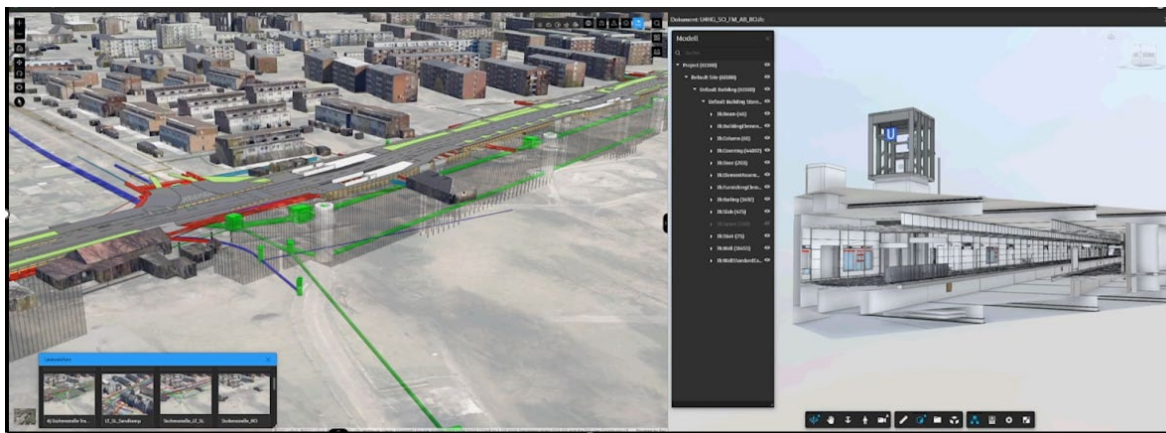
Abb. 3.2.7-2: Integration Gesamtmodell U4 in ArcGIS GeoBIM und Verknüpfung mit BIM360
