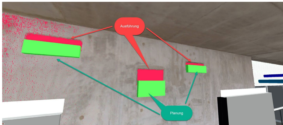
Abb. 3.1.15-3: Obige Fotos: Beispiele einer Abweichung zwischen Planung und Ist-Zustand der Baustelle
