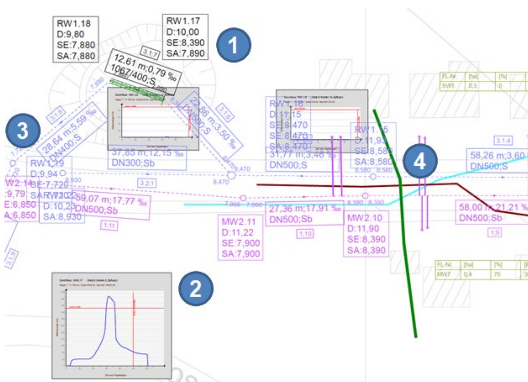
Abb. 3.2.1-2: Ausschnitt Kanallageplan
