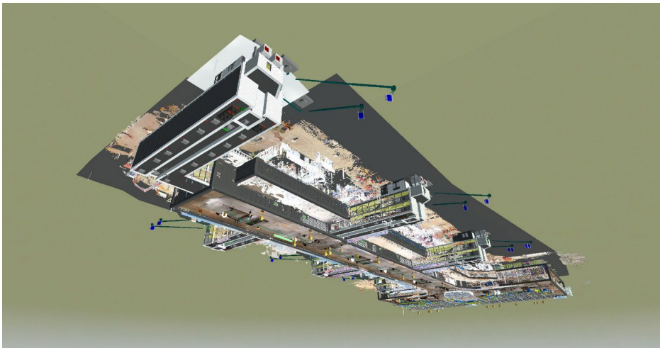
Abb. 3.1.15-2: Vergleich des Scans mit dem BIM-Modell des Terminals
