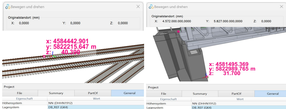
Abb. 3.5.3-3: Exportierte georeferenzierte Koordinaten in IFC mit DB_REF2016 aus einem Trassen-Tool ohne Projektbasispunkt (links) und aus einem Hochbau-Tool mit Projektbasispunkt-Offset (rechts)
