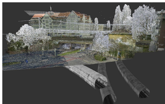
Abb. 3.1.16-4: Ausschnitt Punktwolke terrestrisches Laserscanning + U-Bahntunnel
