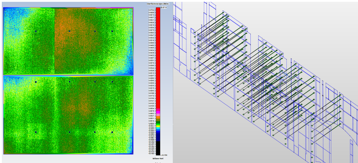
Abb. 3.1.4-2 links: Ergebnis der Punktwolkenanalyse ausgewählter Abschnitte (FARO AS-BUILT für REVIT), rechts: Visualisierte Abstände zwischen Einzelpunkten (DYNAMO-Skript).
