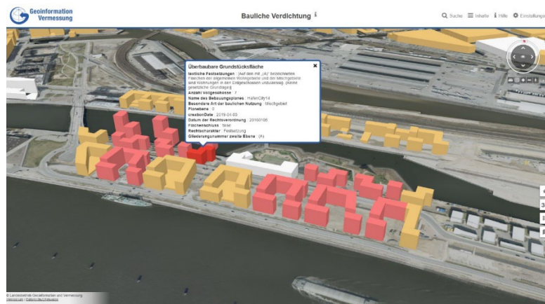
Abb. 2.7-9: 3D-Visualisierung von Festsetzungen eines Bebauungsplans in CityGML.
